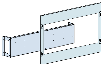
Płyta montażowa W=600 22262
