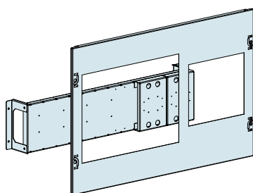
Zestaw płyta + osłona W=800 22846
