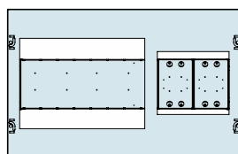
Zestaw płyta + osłona W=800 22846
