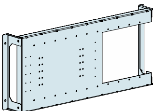
Płyta montażowa W=600 4M 22264
