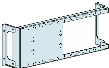
Płyta montażowa W=800 3M 22263
