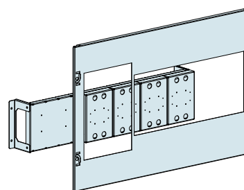
Zestaw płyta + osłona W=800 22845
