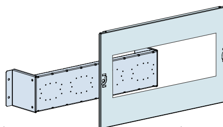
Płyta montażowa W=600 22261
