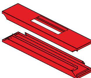
Pokrywy poziome ON D127 - 00164
