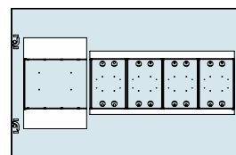
Zestaw płyta + osłona W=800 22845
